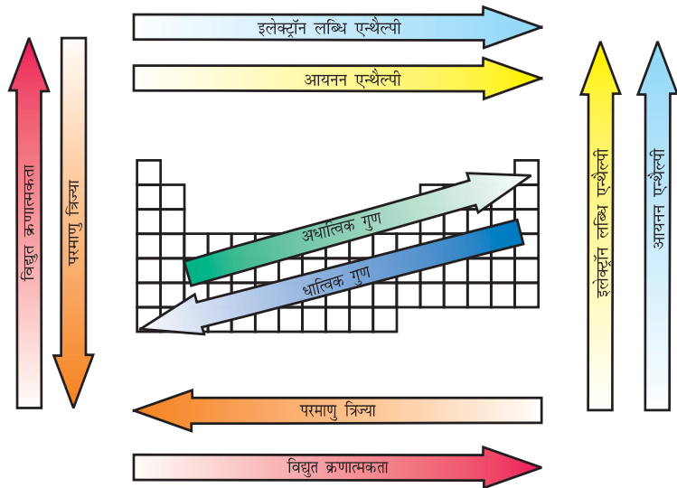
चित्र 3.7 आवर्त सारणी में तत्वों की आवर्त प्रवृत्ति
