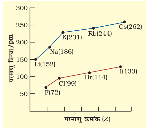
चित्र 3.4 (ख) परमाणु क्रमांकों के साथ क्षारीय धातुओं तथा हैलोजनों की परमाणु त्रिज्याओं में परिवर्तन
