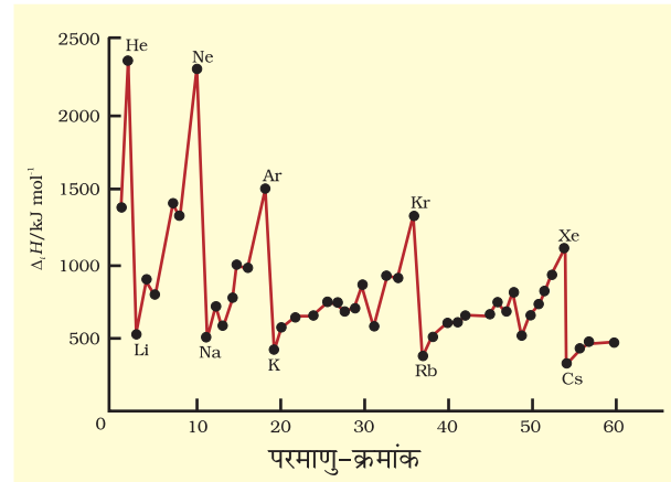
चित्र. 3.5 1 से 60 परमाणु-क्रमांकों वाले तत्त्वों के प्रथम आयनन एन्थैल्पी के मात्रों में परिवर्तन
